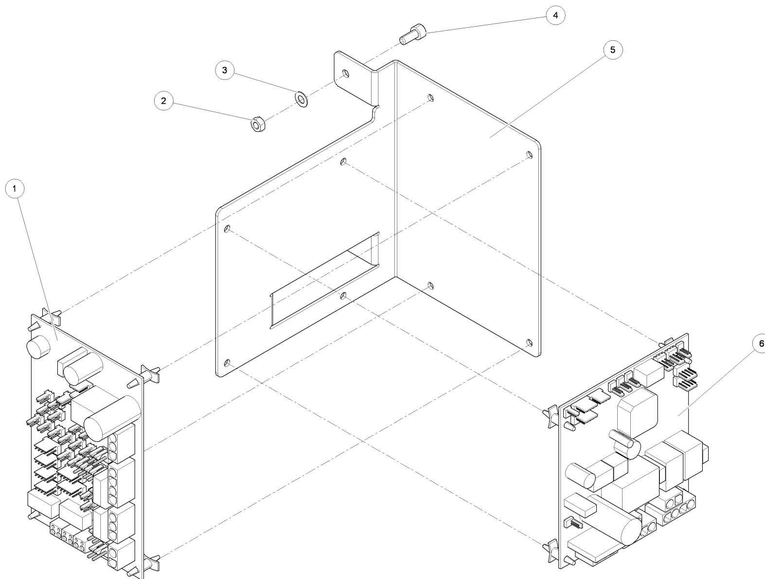
ELEKTROBLOK RIADIACI L - M11783002301
