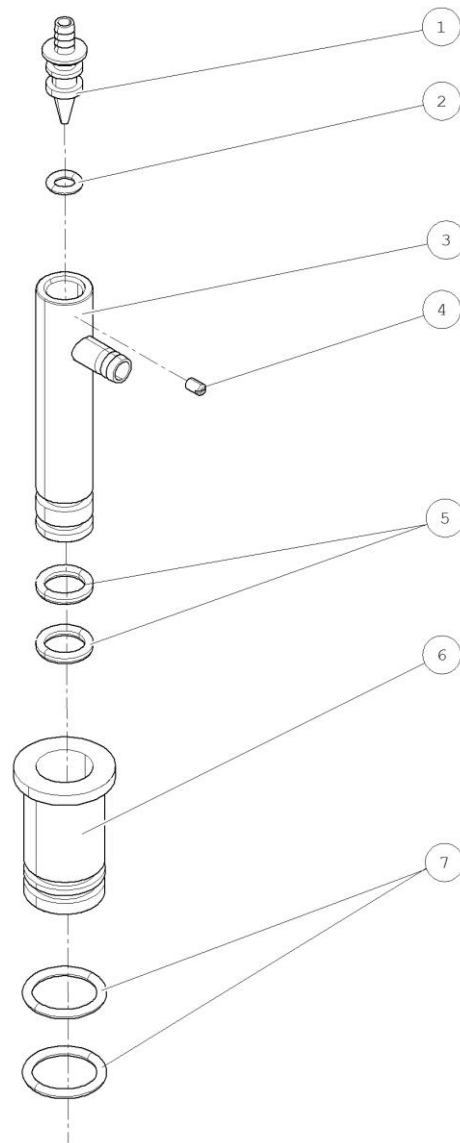
VZDUCHOVY EJEKTOR-MINI - 031274630001
