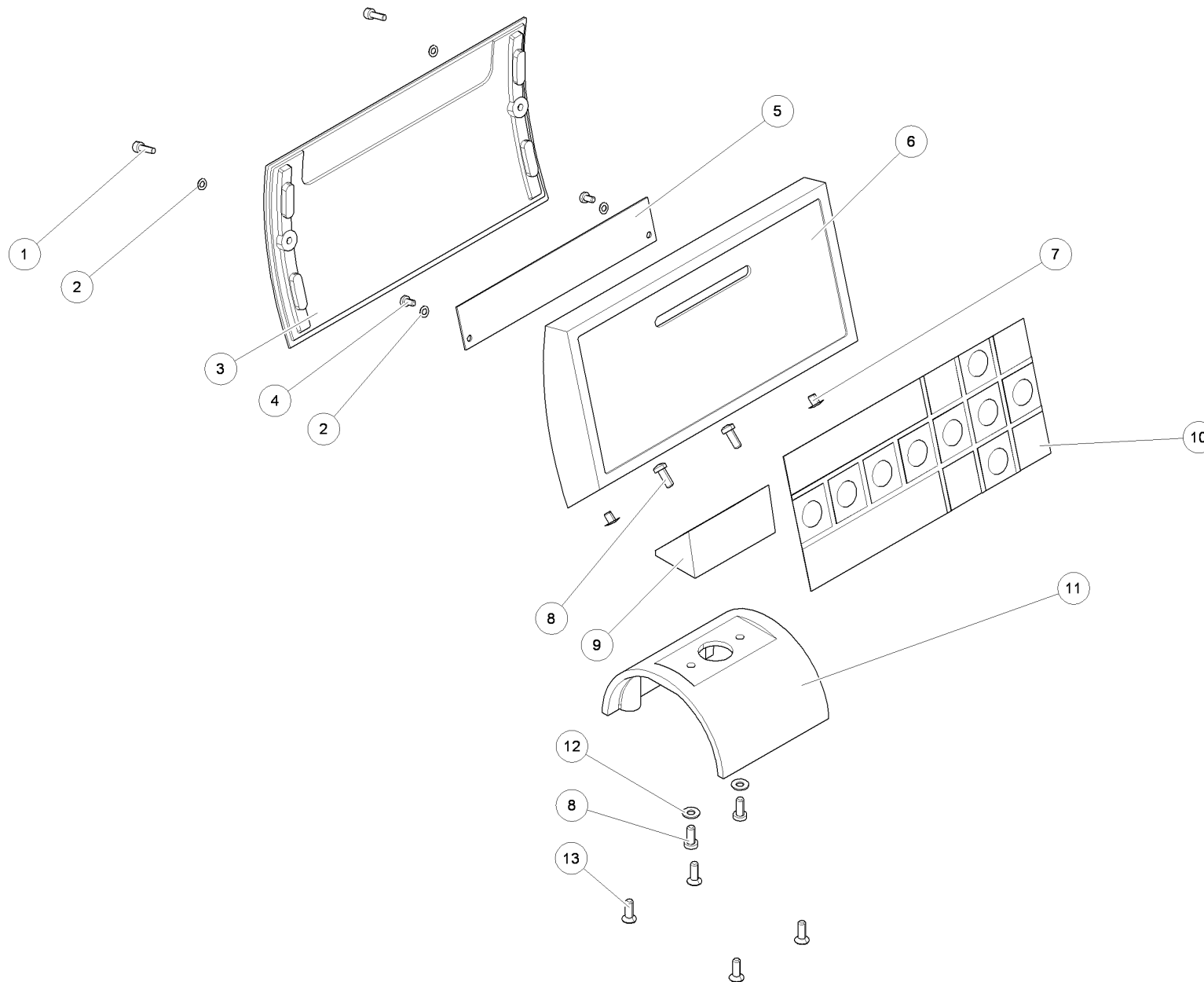
PANEL ASISTENTA 3 - J09197002301
