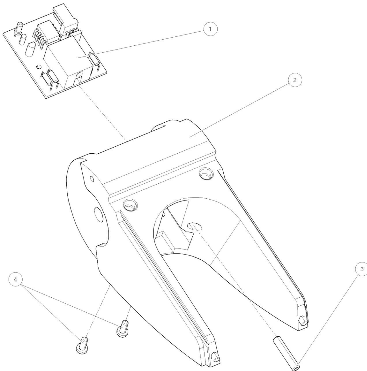
NOSIC DRZIAKA OPTIKA-SL - E08160022301
