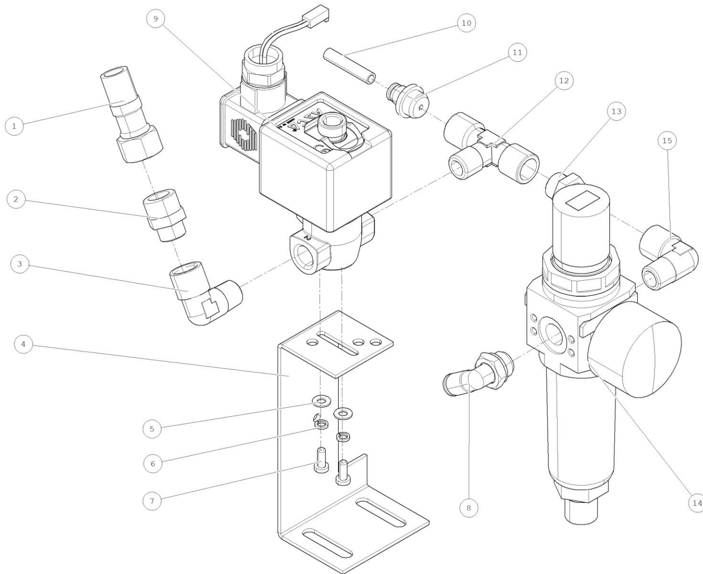
ROZVOD VZDUCHU - V08553002301
