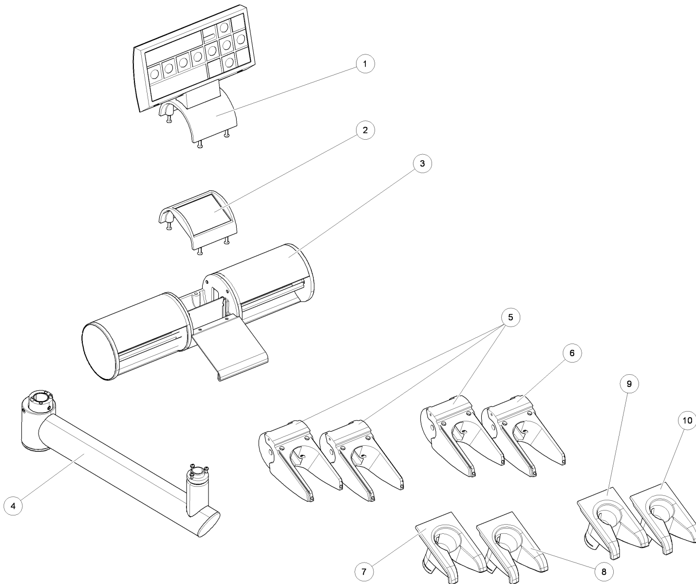
STOLIK ASISTENTA S RAMENOM 4 NASTROJE - J09198002301
