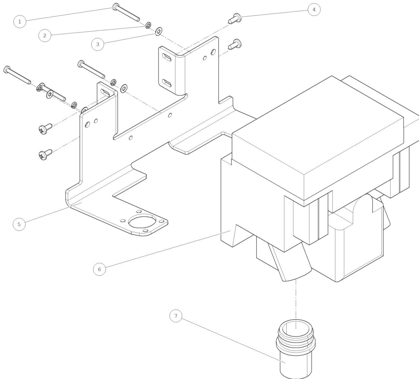
METASYS S1 KOMPLET - V08568002301
