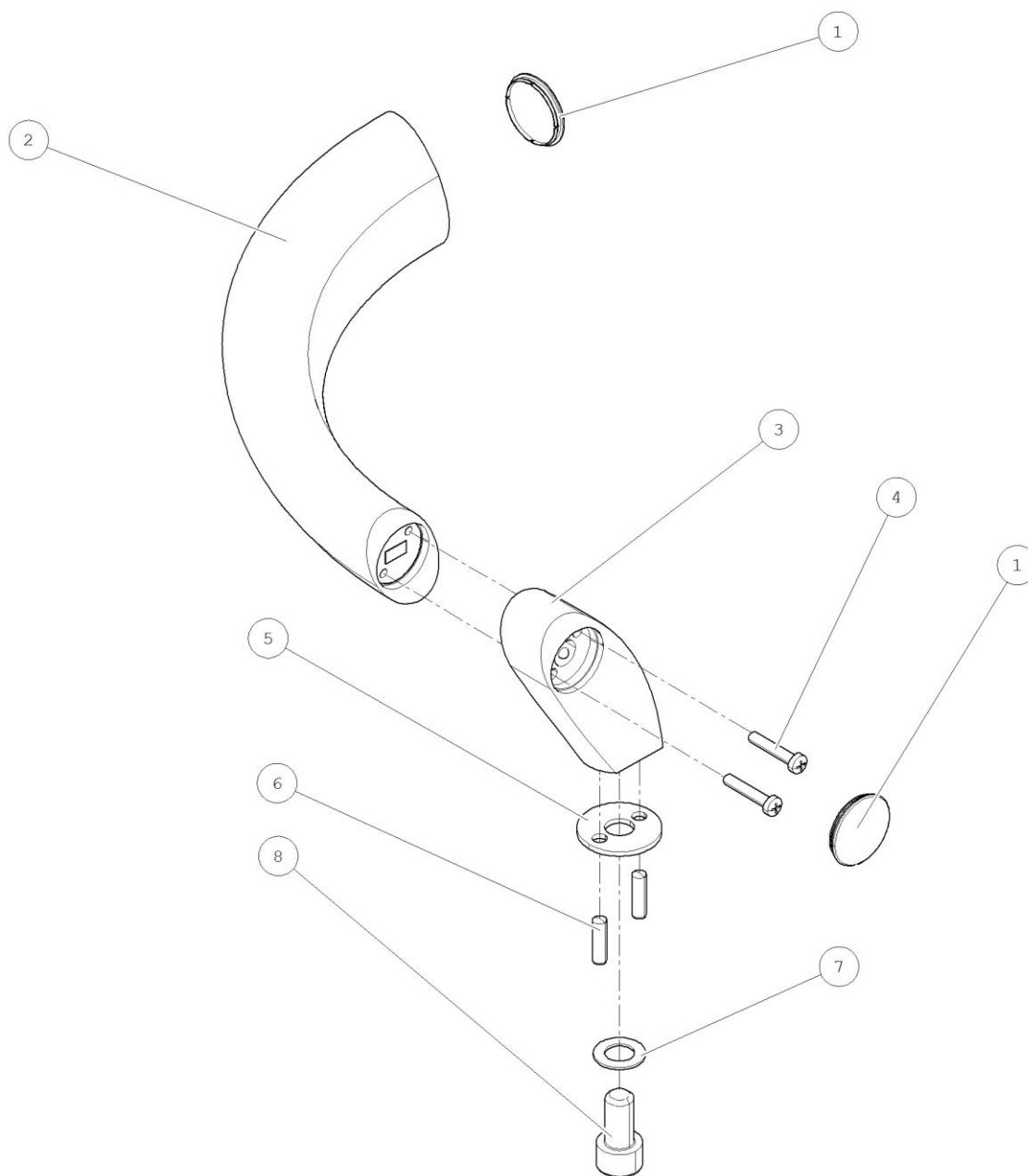
RUKOVAT STOLIKA LEKARA - M08240002201
