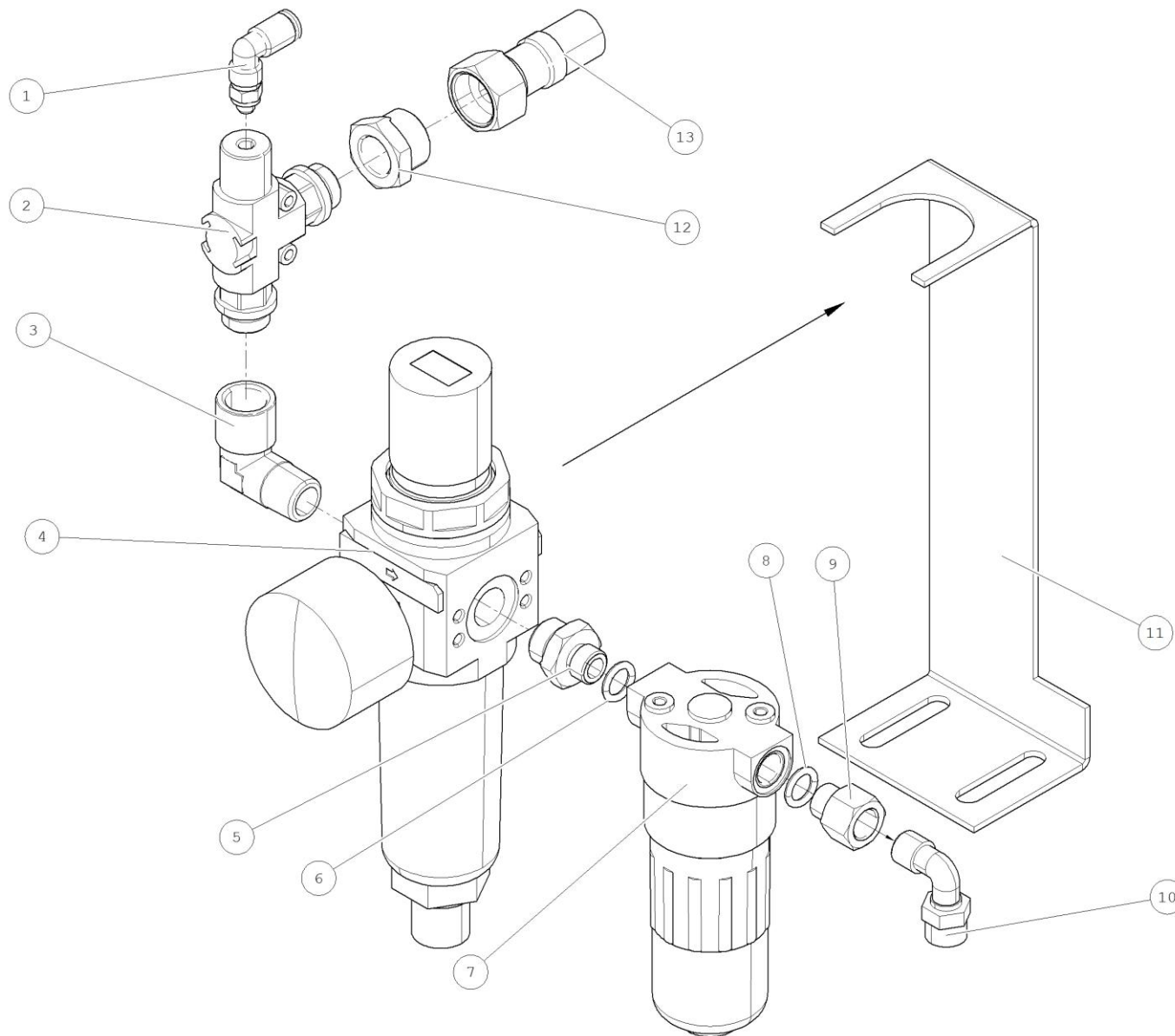
ROZVOD VODY - V08554002301
