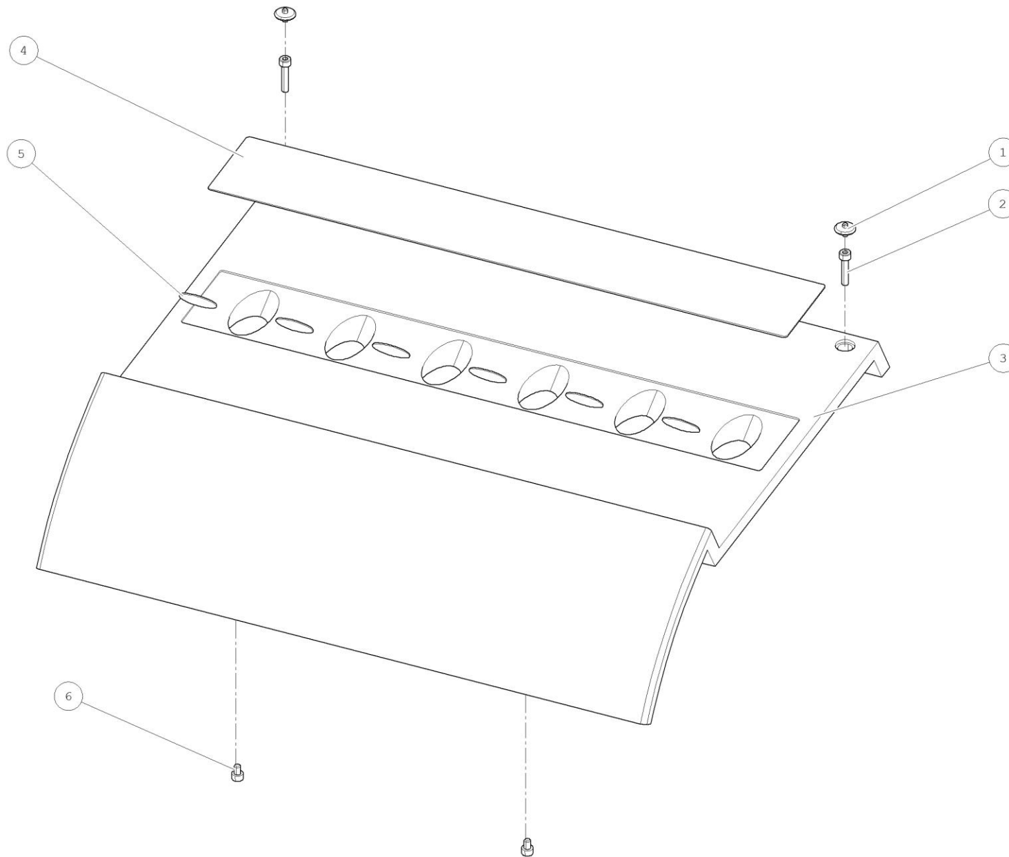
KRYT HORNÝ 6N-DOLNE VEDENIE - E09288012201
