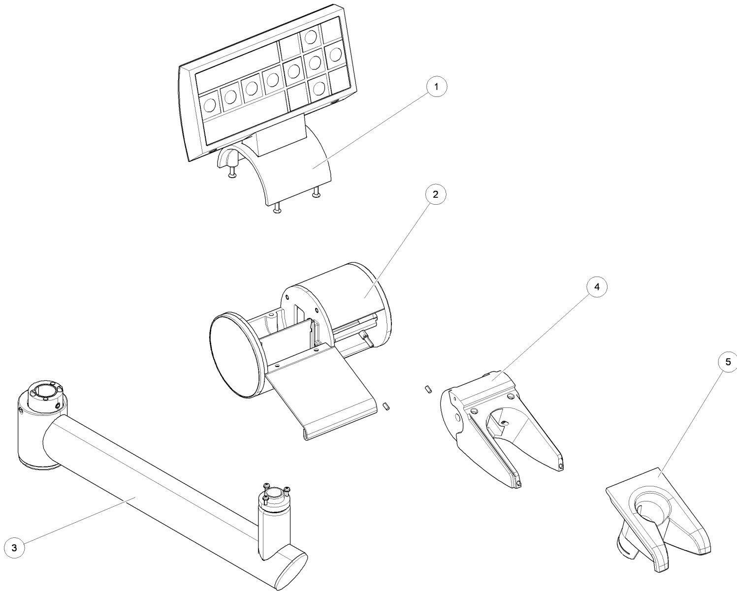
STOLIK ASISTENTA S RAMENOM 1 NASTROJ - J09198002301
