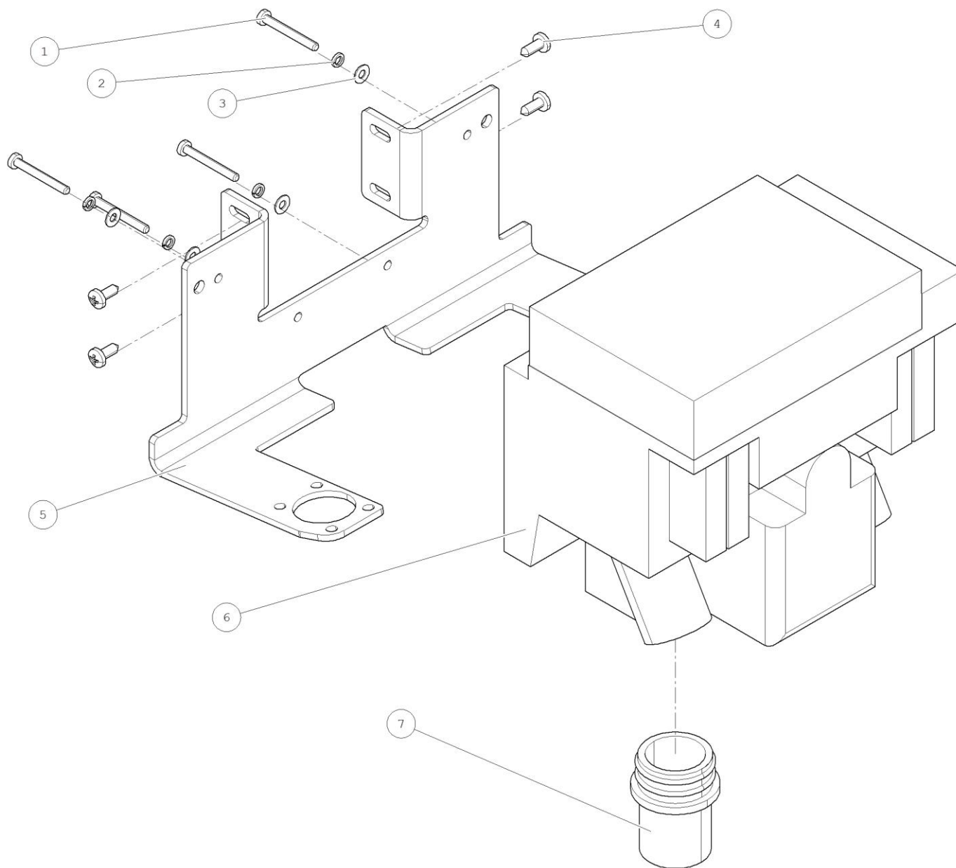
METASYS H1 KOMPLET - V09691002301
