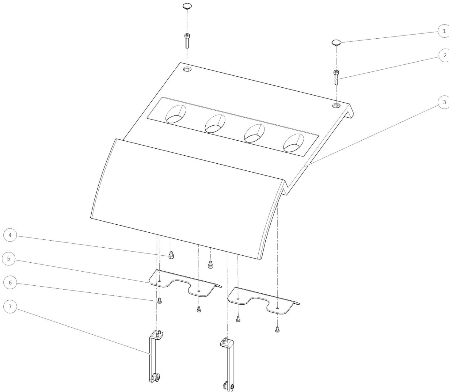
KRYT HORNY 4N-HORNE VEDENIE - E09287022201
