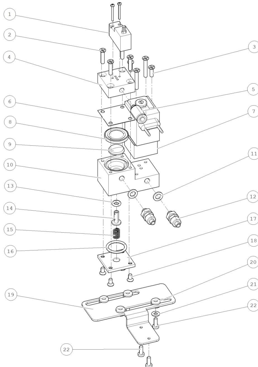
BATERIA W - J08083002201
