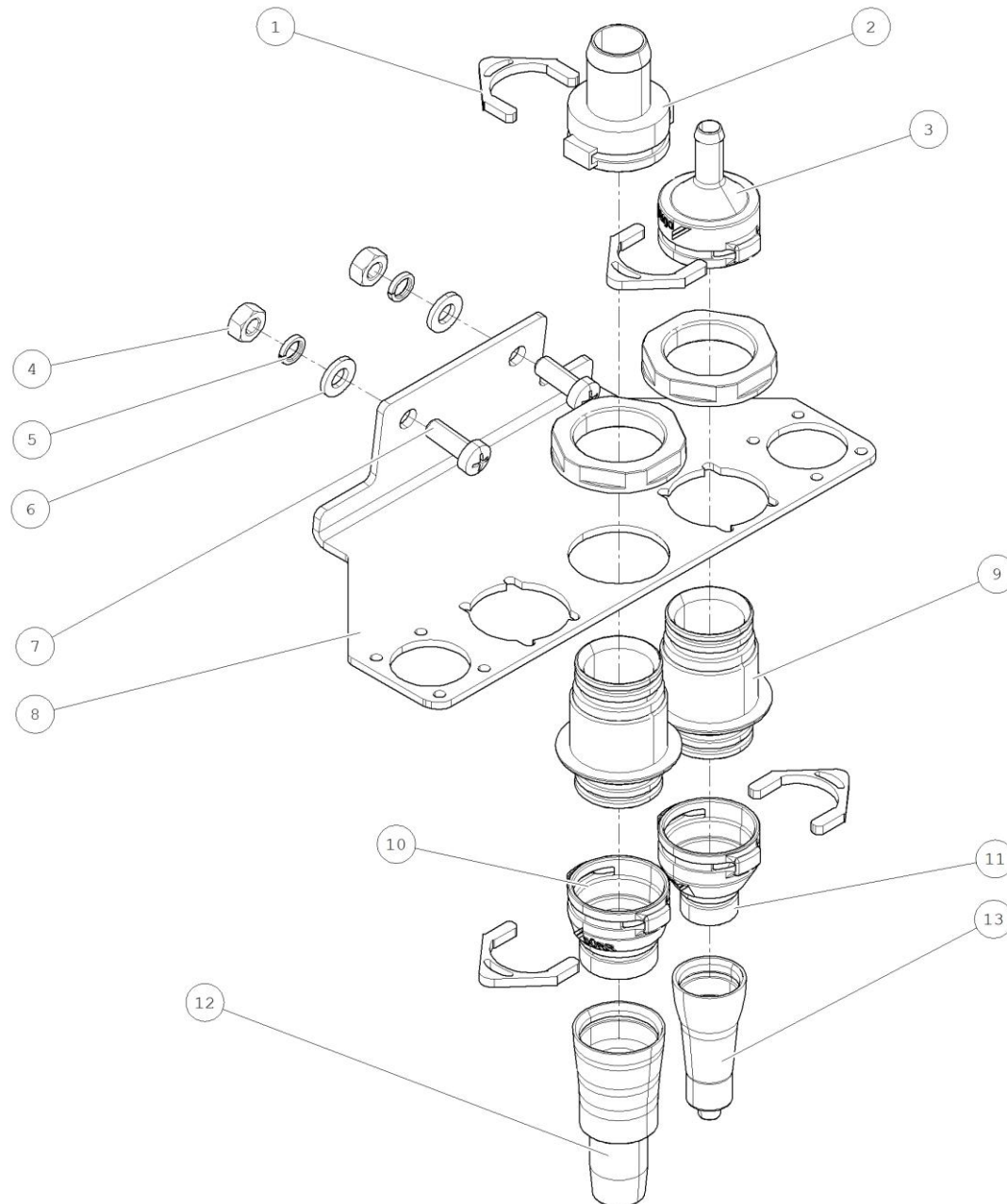
DRZIAK HADIC EJEKT. S 2x HADICAMI - V08536002301
