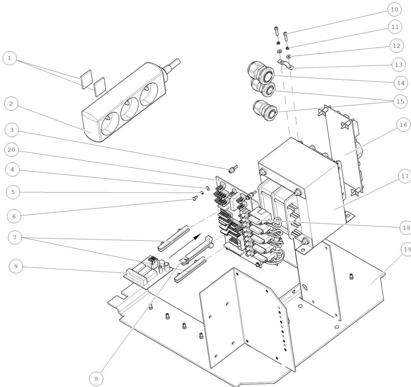
SKRINA PRIVODNA-ELEKTROBLOK - V08523002201
