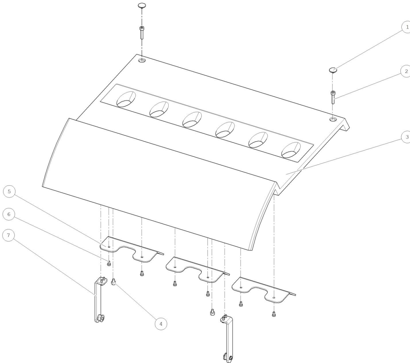
KRYT HORNY 6N-HORNE VEDENIE - E09288022201
