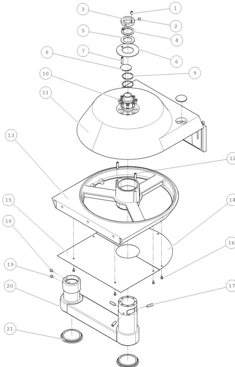
STOLIK ZAKLAD PRAVY - E09259012201
