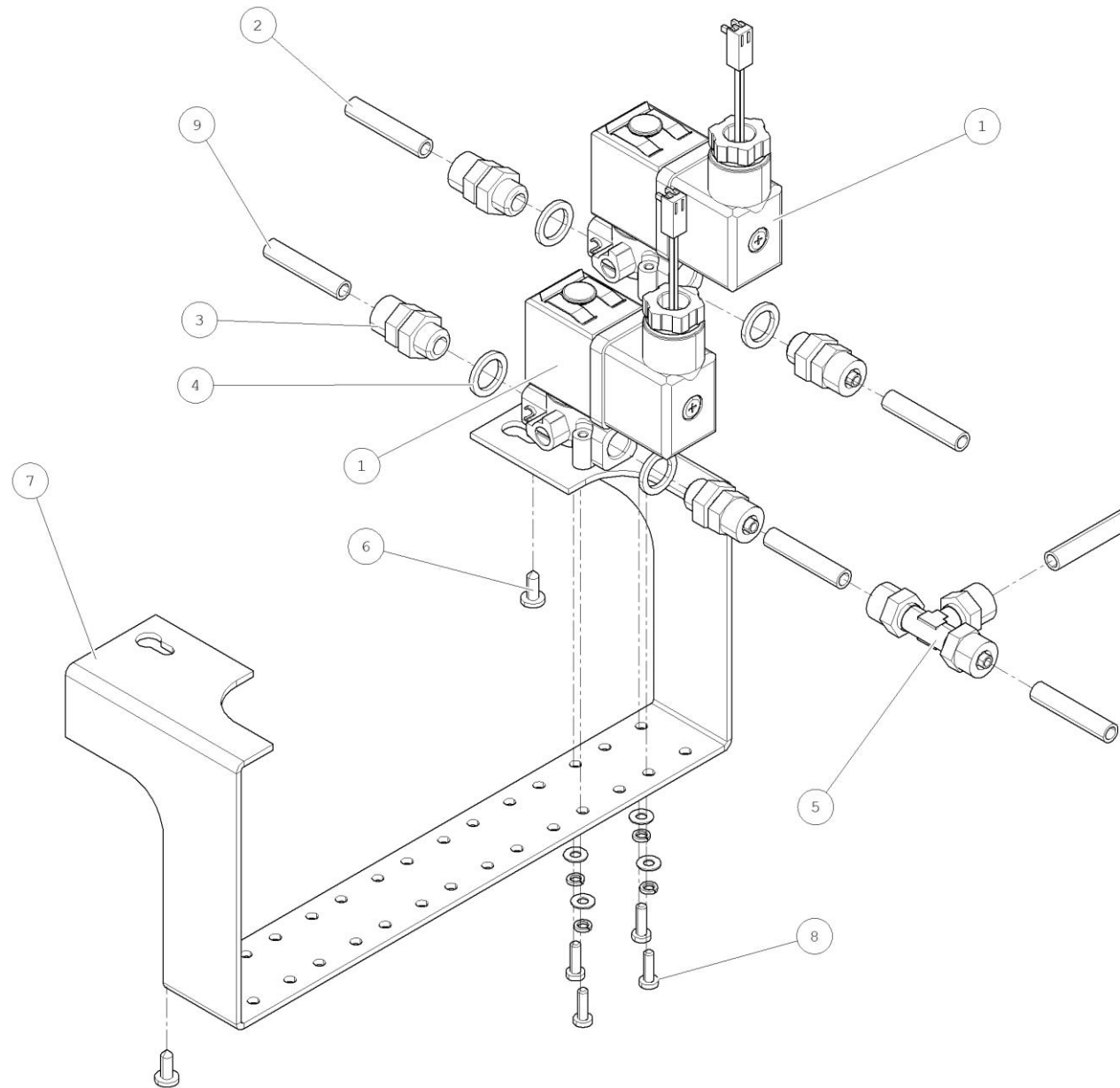
ROZVOD VODY (STUDENA+TEPLA) - V08564002301
