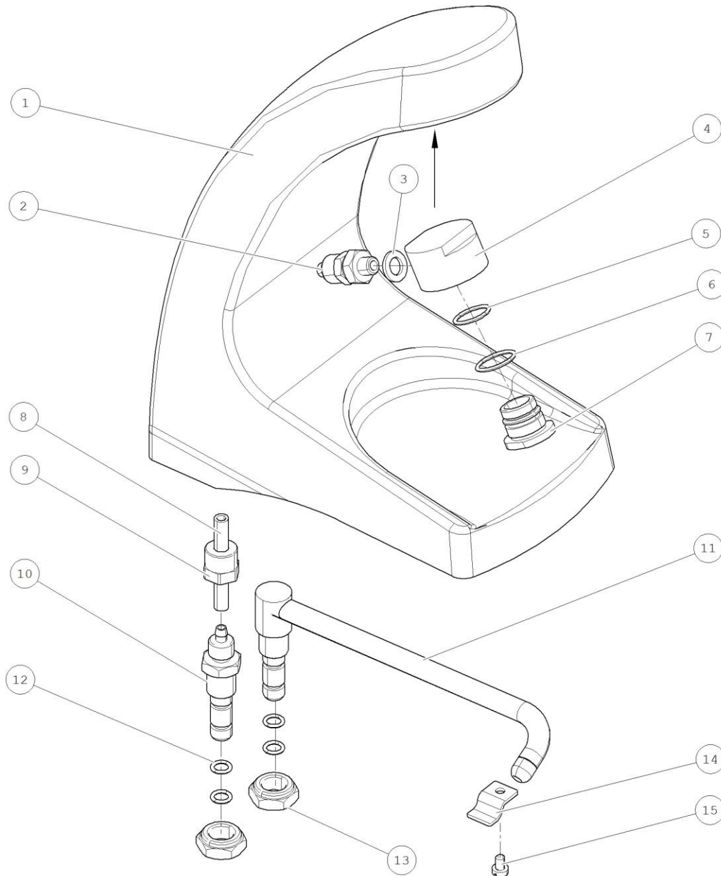
SPRSKA KOMPLET - M08200002300
