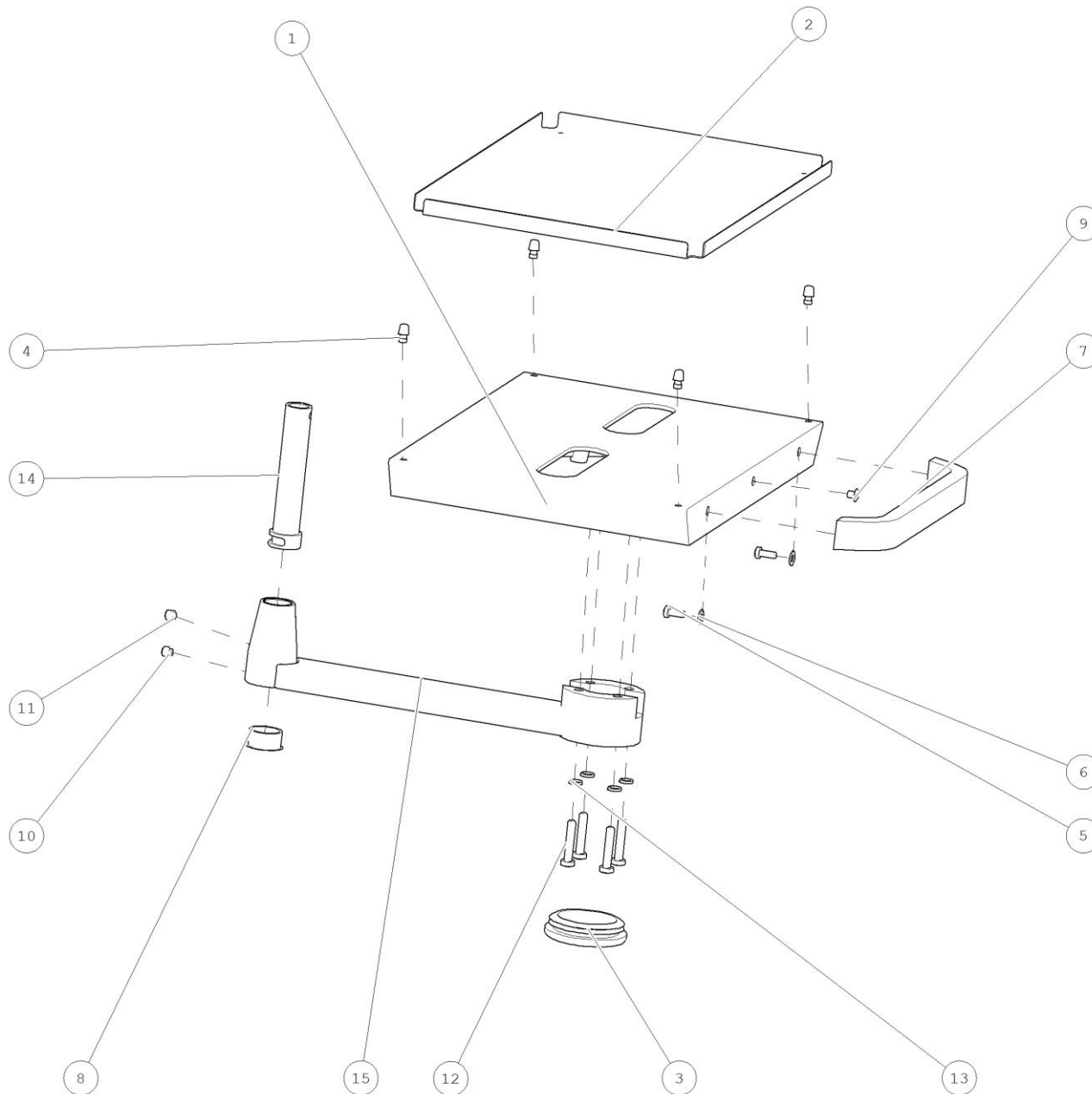
TRAY STOLIK - C09 - 1910022
