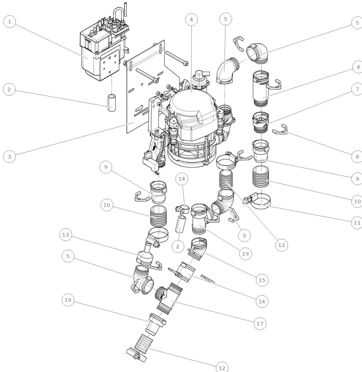
DURR CS1 S VYPLACHOVOU JEDNOTKOU - V09684002201
