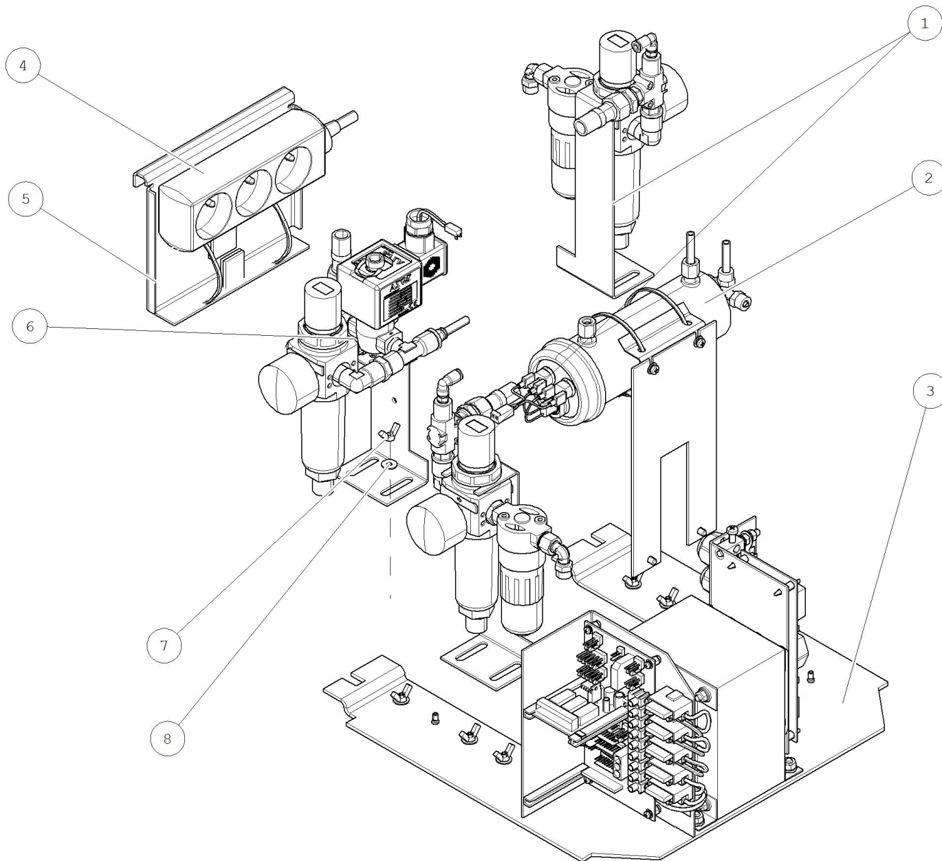
SKRINA PRIVODNA - V08525002201
