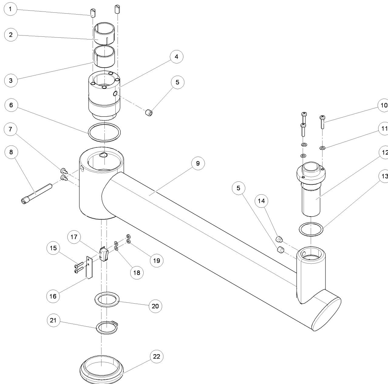
RAMENO ASISTENTA L=330 - C09211002202
