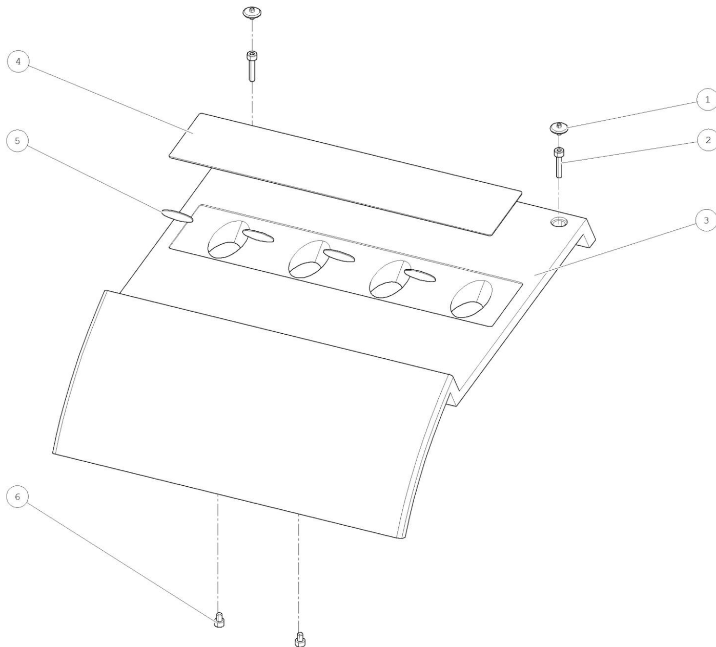
KRYT HORNÝ 4N-DOLNE VEDENIE - E09287012201
