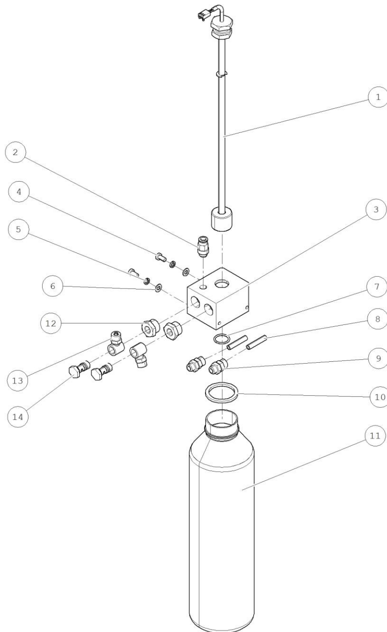
ZASOBNIK MEDIA - V08547002300
