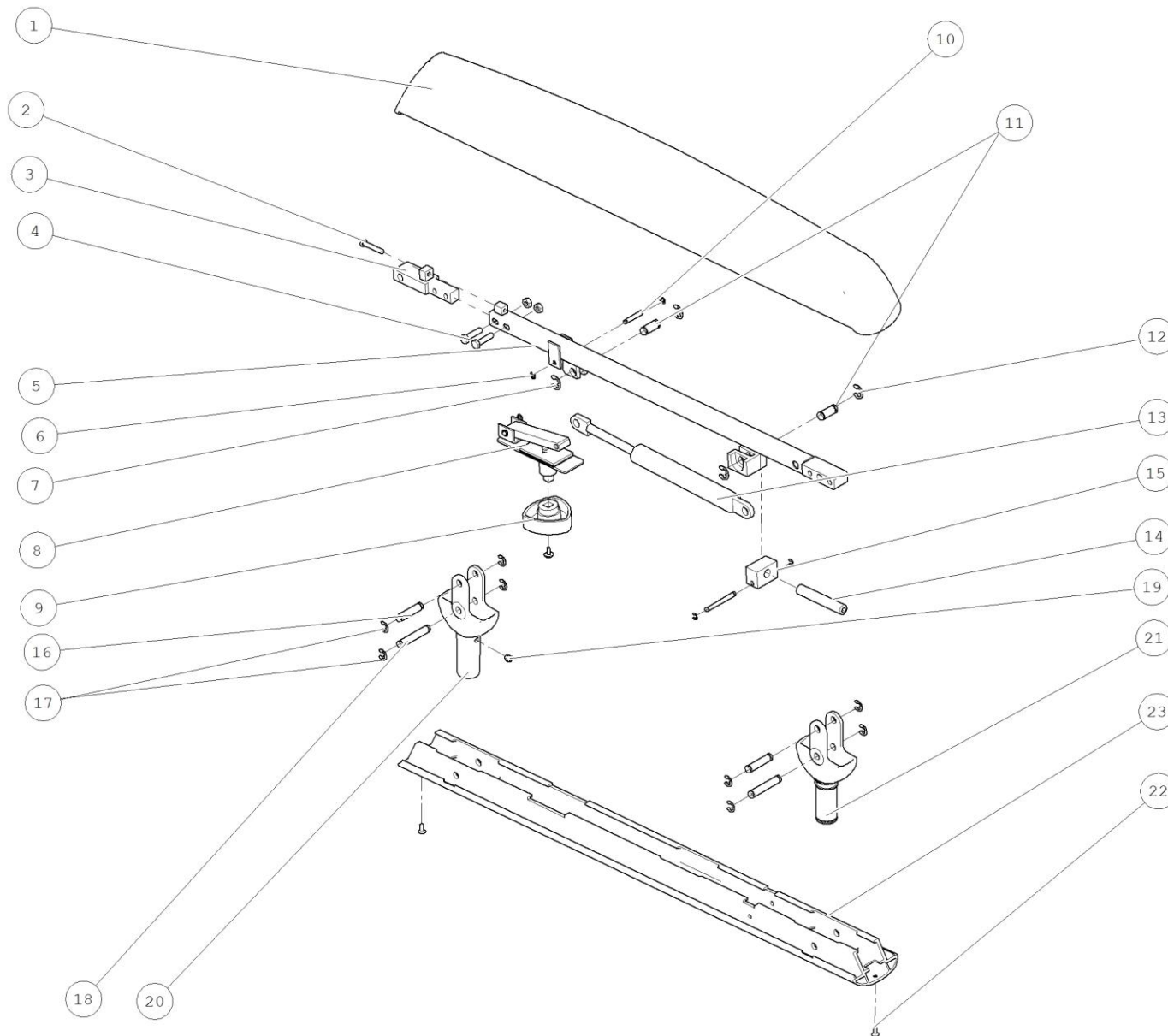
PANTOGRAF TACKY - C08-091002201
