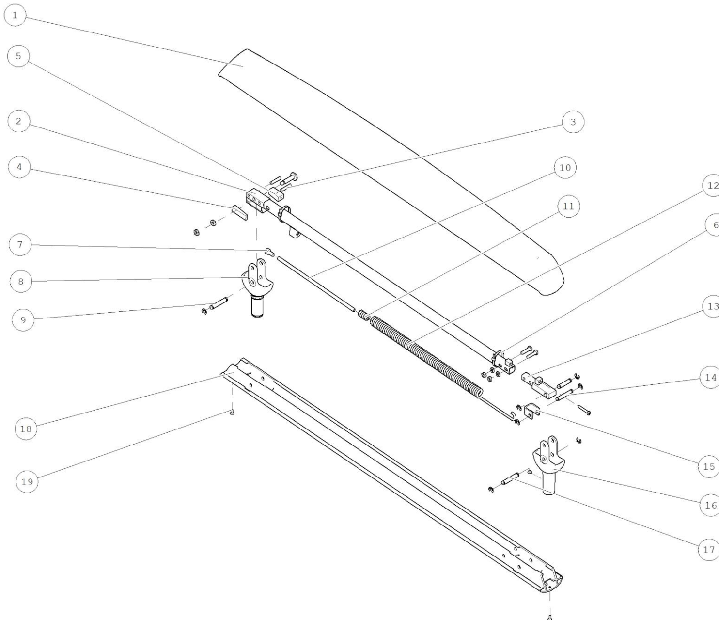
PANTOGRAF SVIETIDLA - C08-08000
